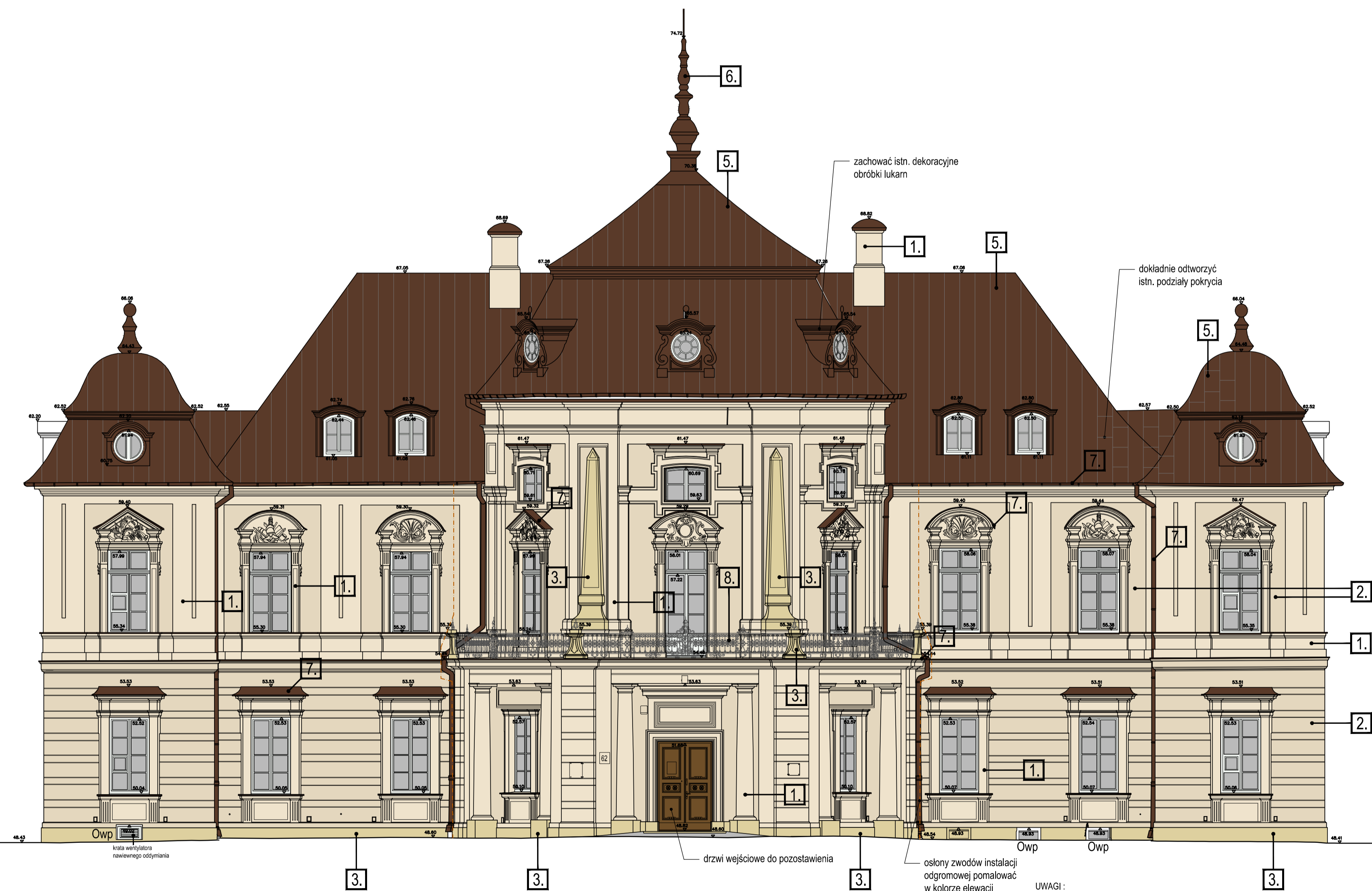
ELEWACJA ZACHODNIA
