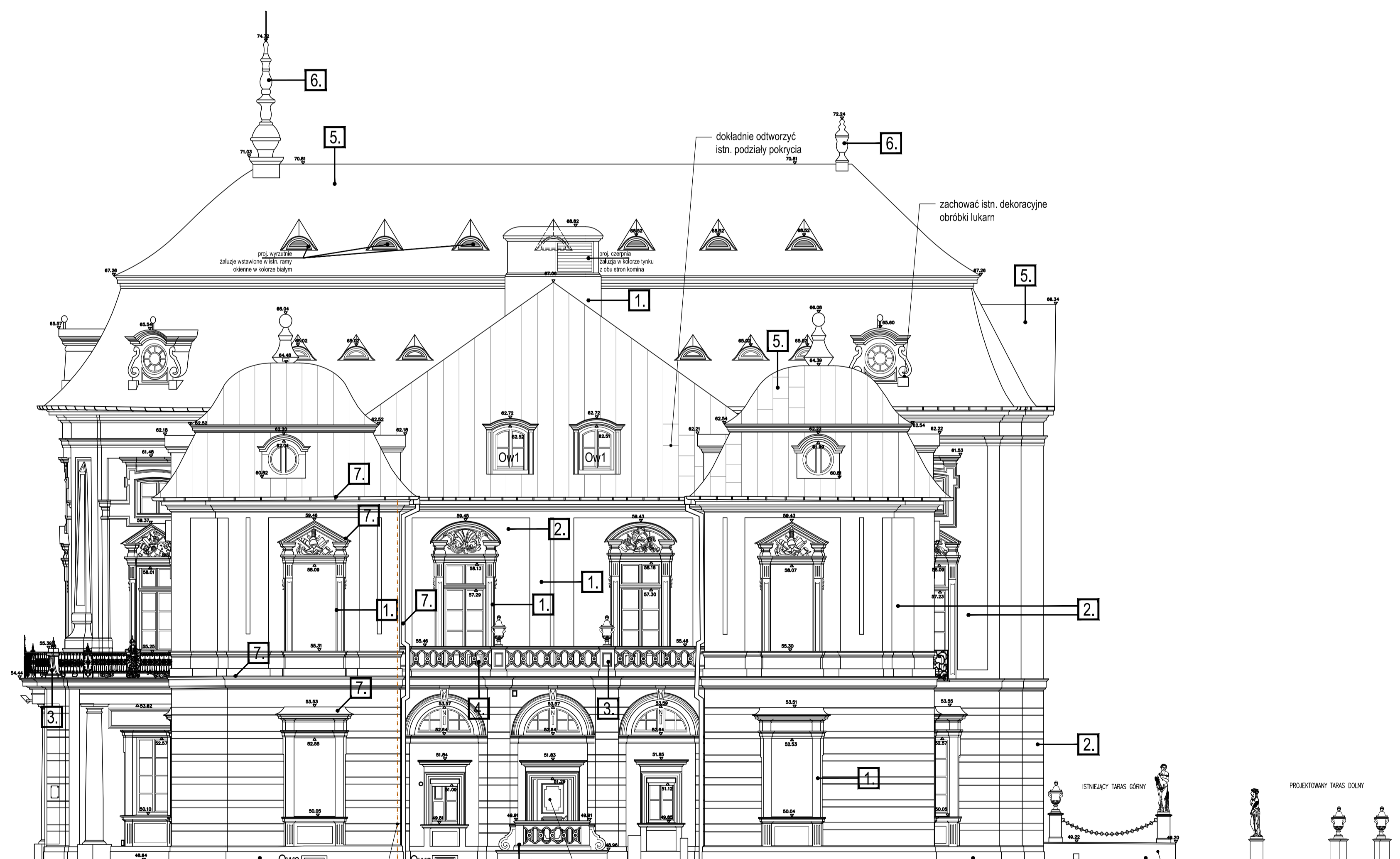
ELEWACJA POŁUDNIOWA
